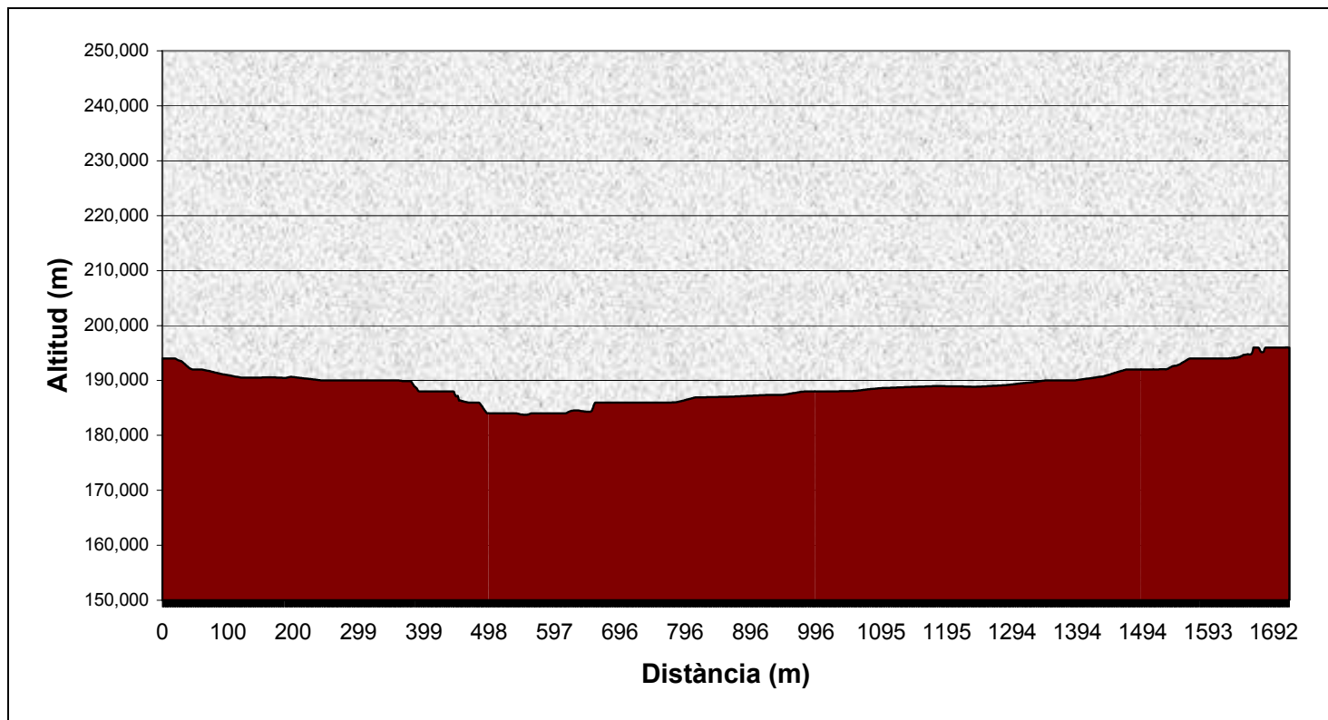
Perfil longitudinal del Camí de la Bleda
