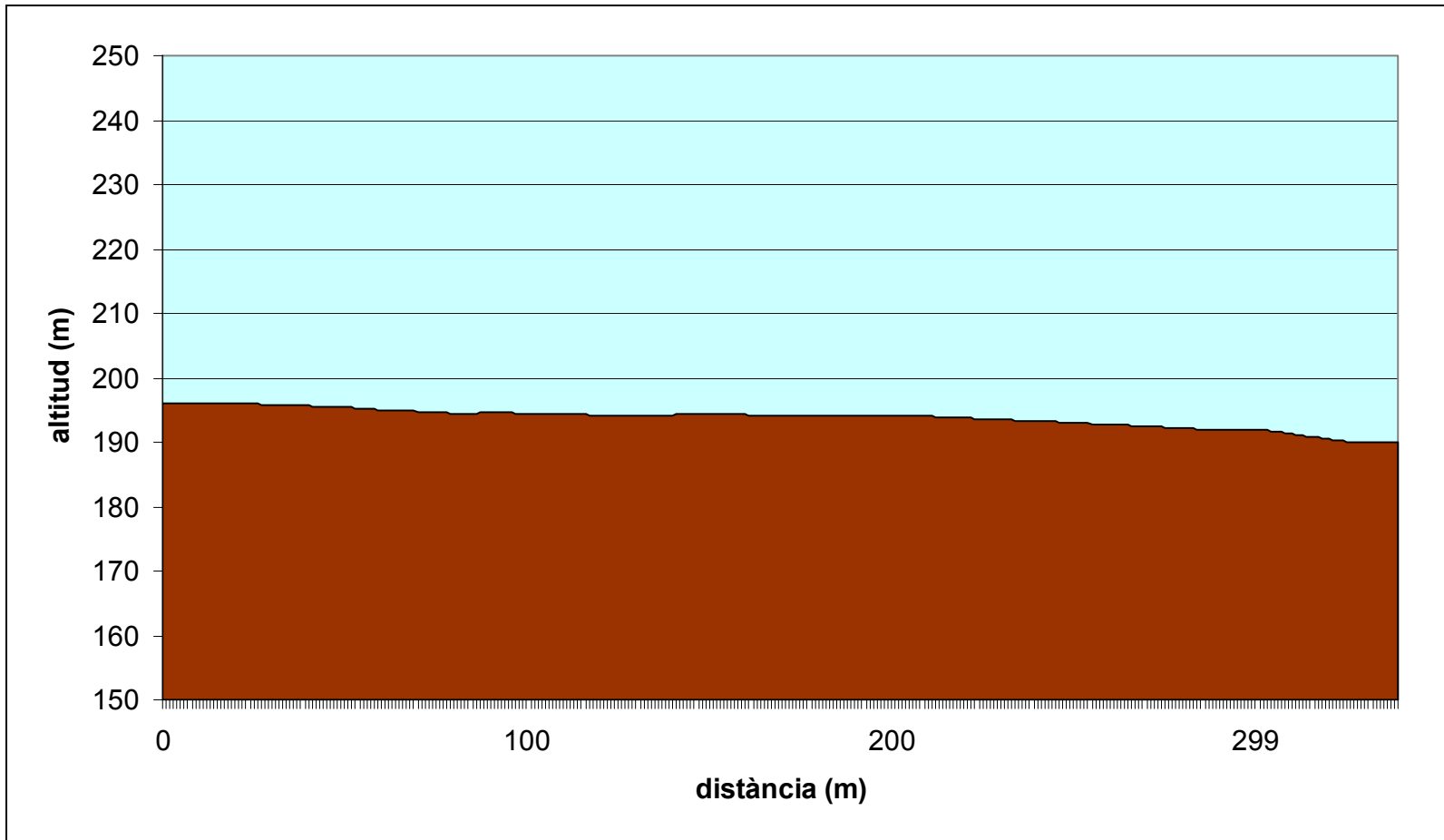
Perfil longitudinal del Camí d'enllaç entre Ciutat Jardí i el camí Fariner
