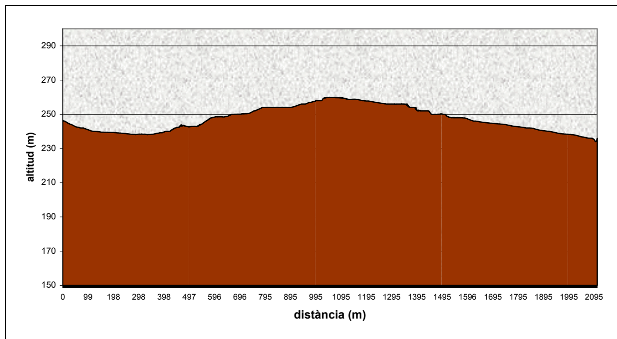
Perfil longitudinal del camí de la Torreta dels Bous
