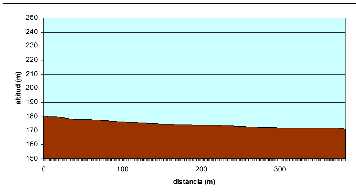
Perfil longitudinal del Camí de Cal Salines
