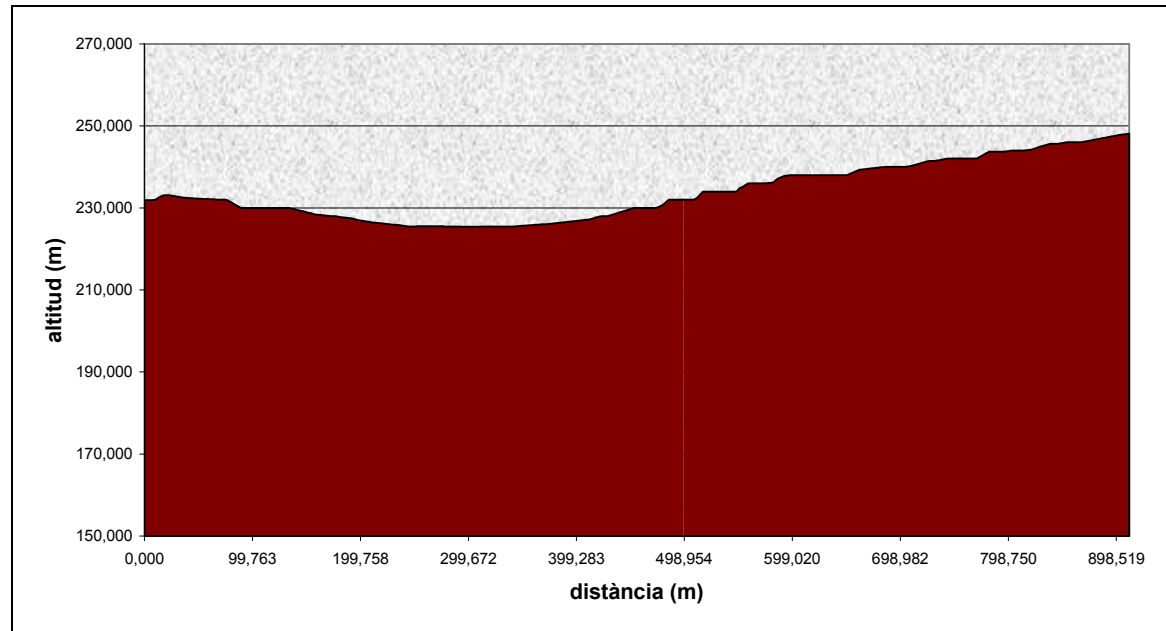
Perfil longitudinal del camí Creu de la Pelegrina.
